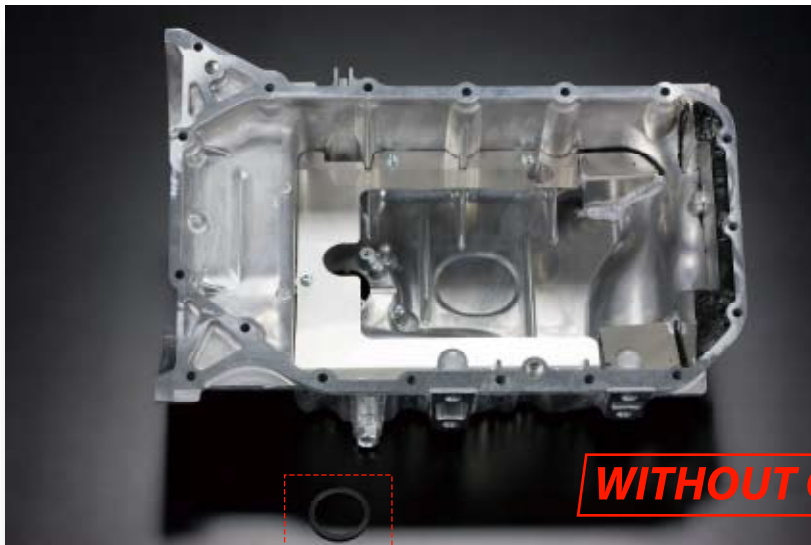
アンチ G フォース オイルパン K20Z FN2 用
