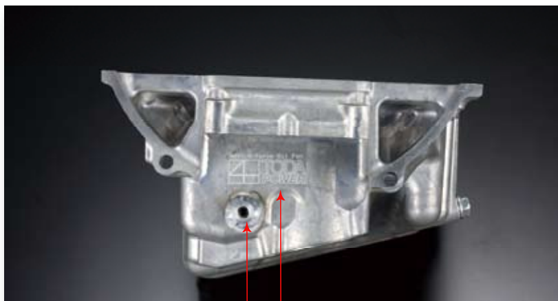
油温計 1/8 PT 取出口 TODA Mark
